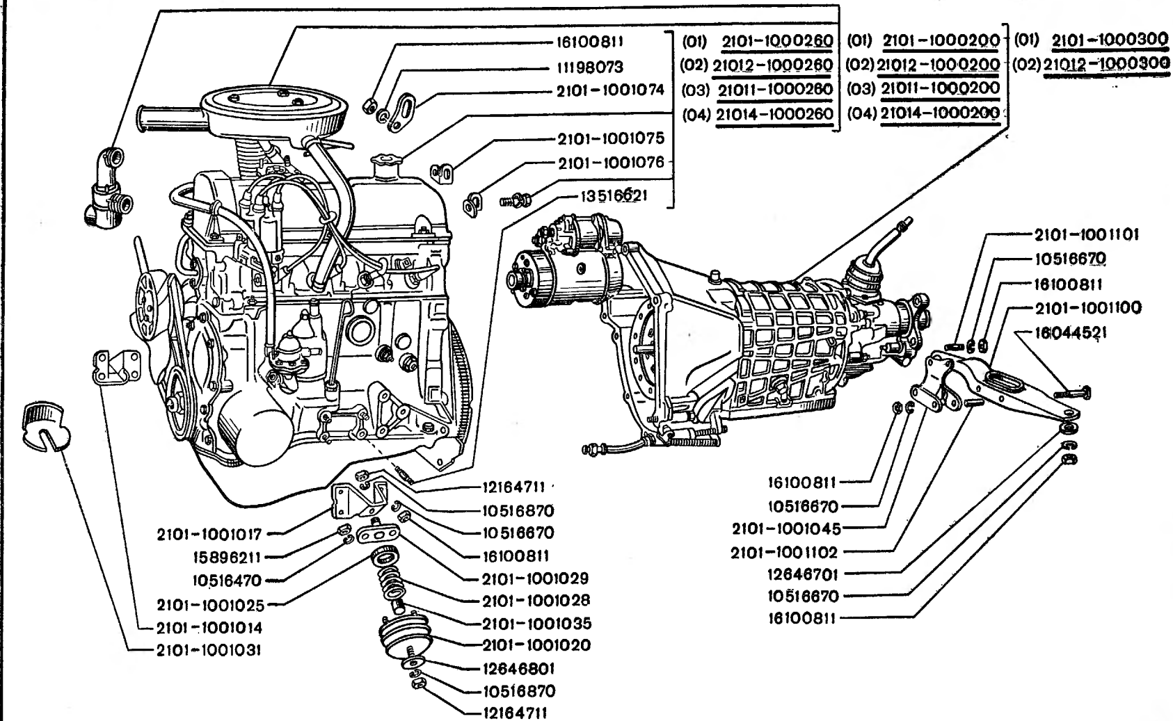
ДВИГАТЕЛЬ И ПОДВЕСКА ДВИГАТЕЛЯ
