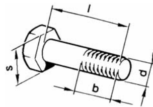
Болт с шестигранной головкой
