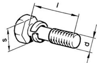
Болт с пружинной шайбой
